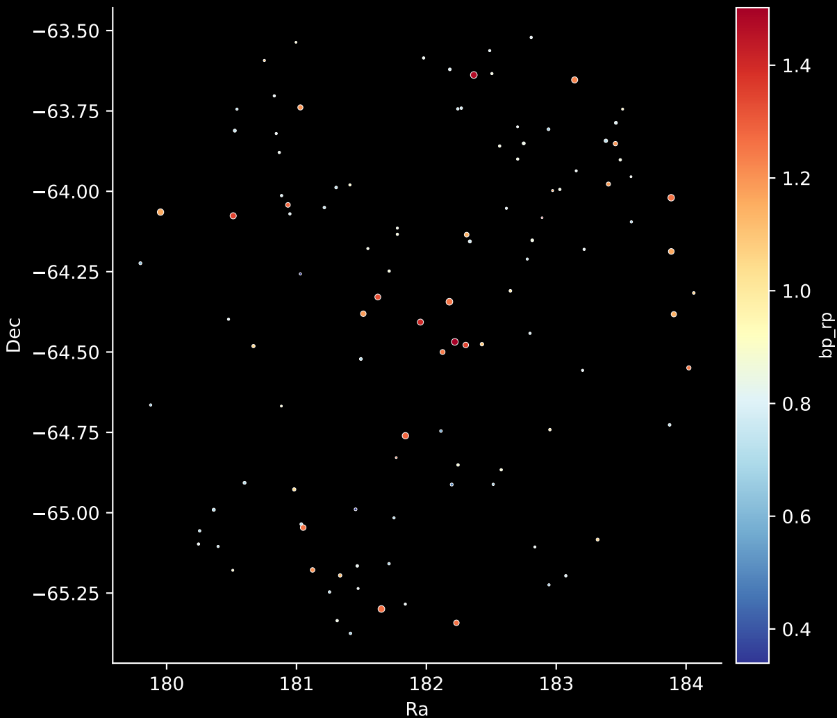
GALAH DR4 Field: [7125] Stars: 110
