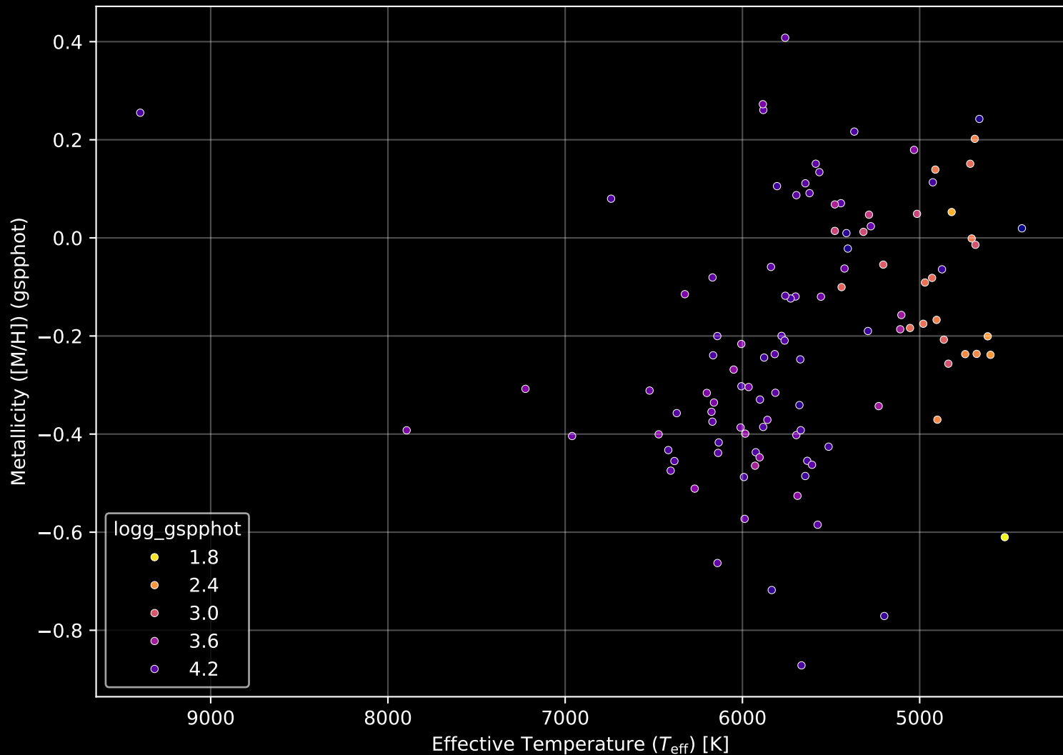
GALAH DR4 Field: [7125] Stellar Population Parameters (n= 110)
